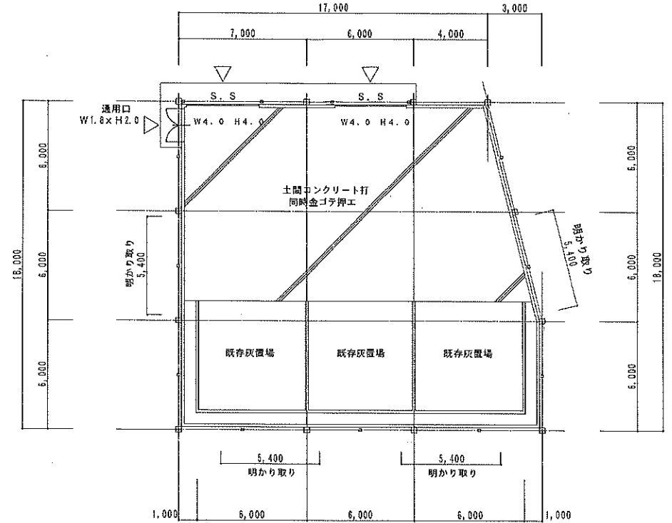
灰置場 平面図 S=1/200
